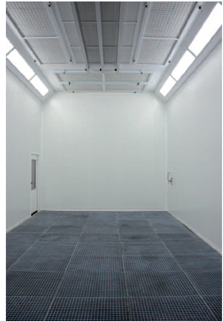
Die Belüftung der beheizbaren Nasslackkabine ist mit einer Wärmerückgewinnung kombiniert.
